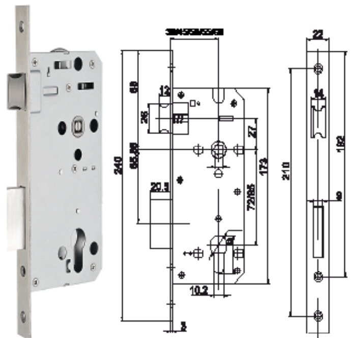
Serratura Antipanico Europea 6085/6072 da infilare
