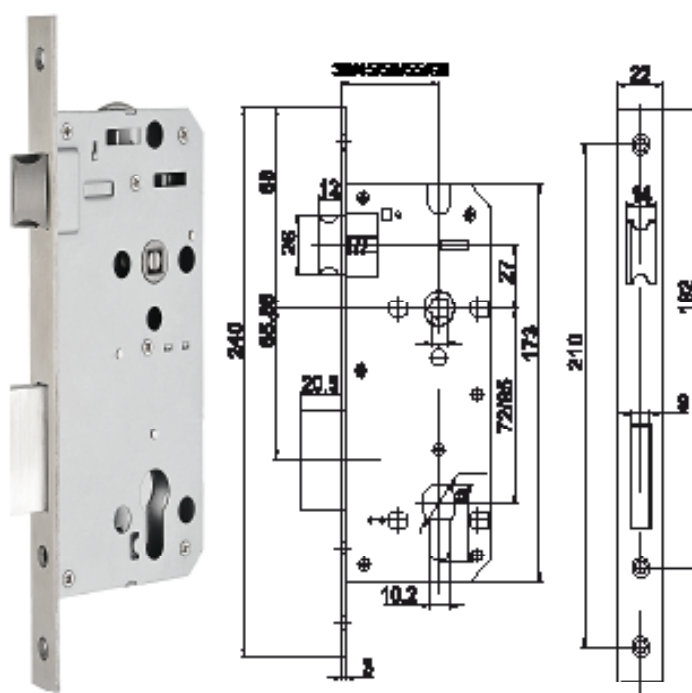
Serratura Antipanico Europea 6085/6072 da infilare
