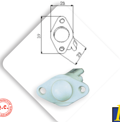
RB34C - SENSORE STATO PORTA A BIGLIA
