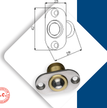
BALLCONTACT - SENSORE STATO PORTA
