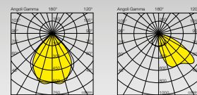
mod.PR ottica simmetrica 90° mod.AR ottica asimmetrica 45°
