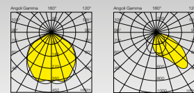
mod.P9 ottica simmetrica 90° mod.A5 ottica asimmetrica 45°
