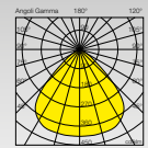
mod.S5 ottica diffusa 90° UGR<25
