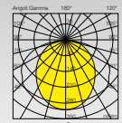
mod.LD ottica diffusa 120°
